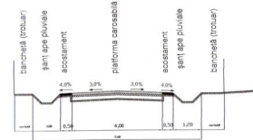
Seciune caracteristică strazi reabilitate, 4,00 m
